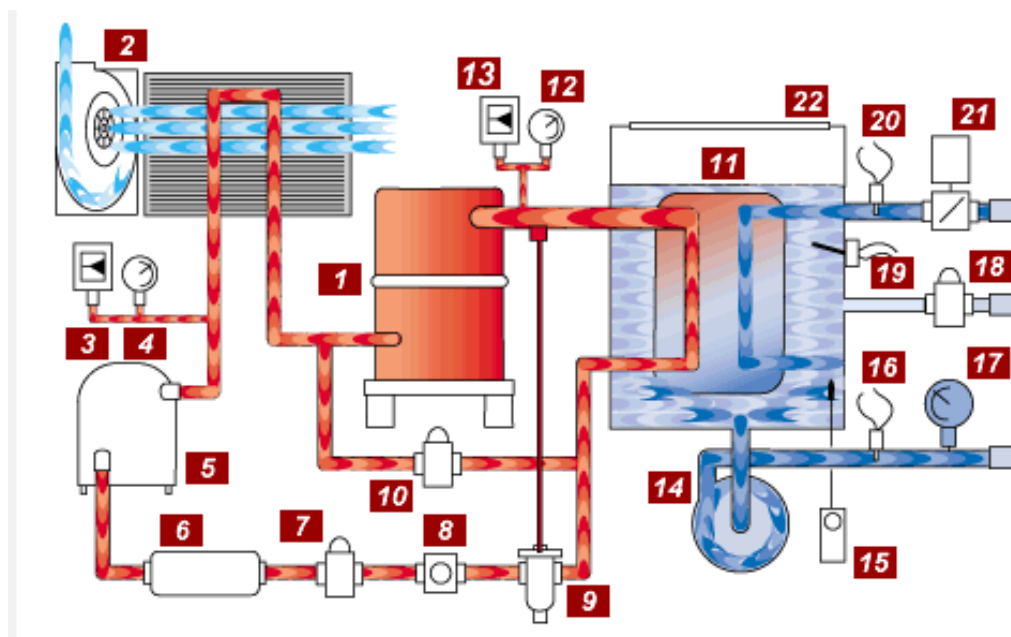
1. attēls. Gaisa kondicionēšanas sistēma (chiller)
