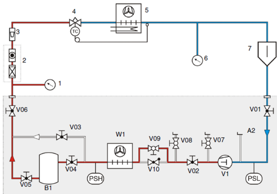
1. attēls. Saldēšanas sistēma
